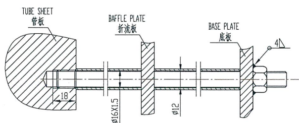
TIE ROD DRAWING 拉杆结构图
