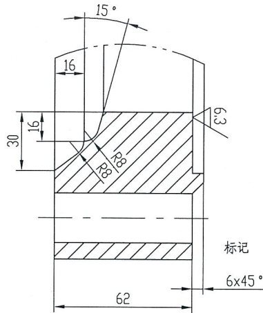
DETAIL DRAWING OF SECTION I I 部详图 NO SCALE 不按比例
